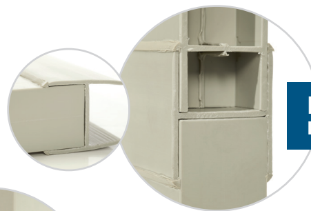
U-PROFIL z PP k připojení panelů a zakrytí otevřených komor
